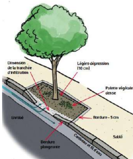
Schéma de principe de l'intégration d'une fosse d'arbre dans un aménagement de voirie.
