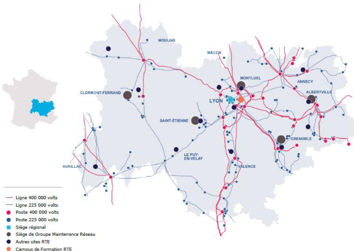
Figure 2 - Carte du réseau 400 et 225 kV en Auvergne Rhône-Alpes
